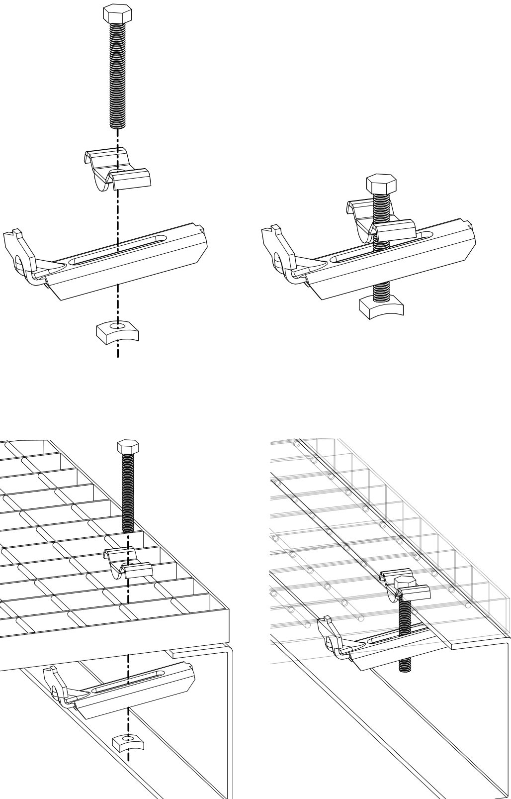
Montering av komplett fästdetalj till gallerduk. Princip visar H-durk och U-balk.
