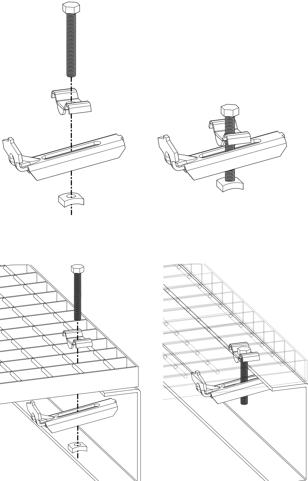
Montering av komplett fästdetalj till gallerdurk. Princip visar H-durk och U-balk.
