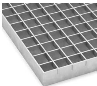
A22X22 Maskvidd: c/c 22x22 mm
